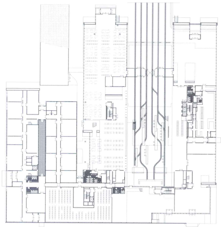
图书馆一层平面图
