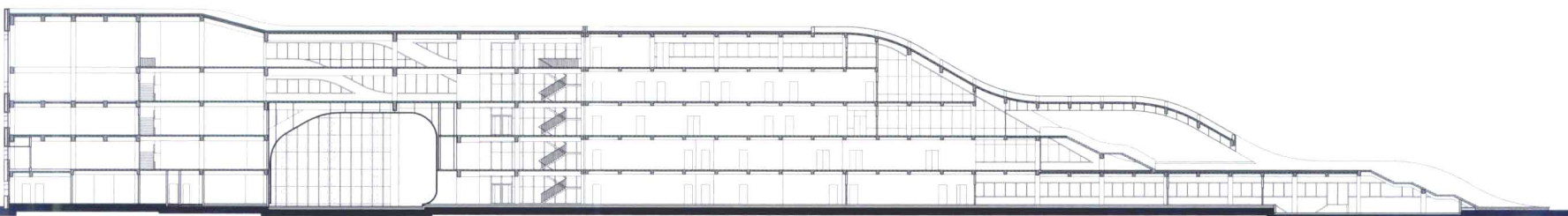
少年宫剖面图
