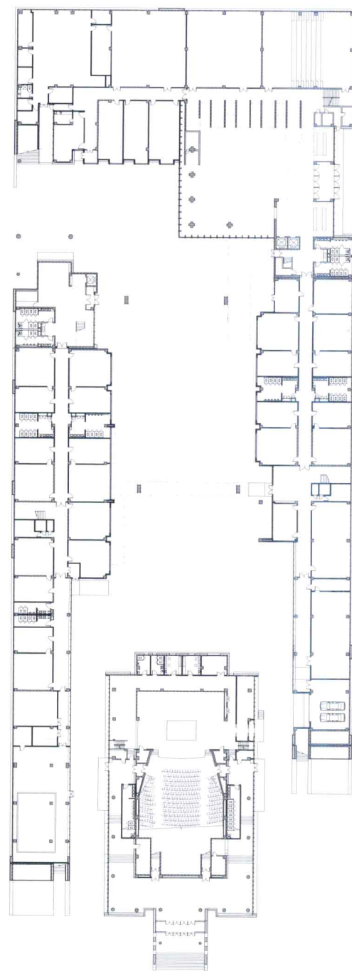
少年宫一层平面图
