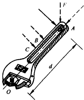
图 1-9 力矩
