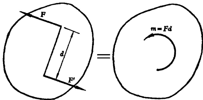
图 1-14 力 偶矩
