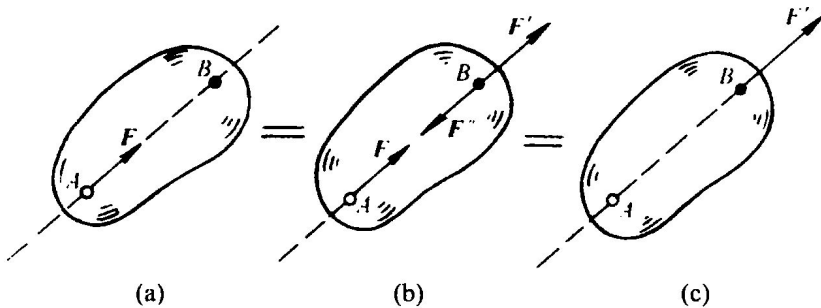
图 1-4 平衡力系
