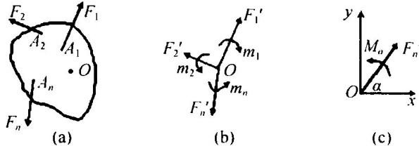
图 1-18 刚体受力简化示意图
