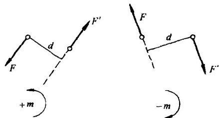
图 1-11 力偶与力偶矩的简化图
