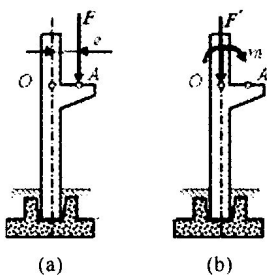
图 1-16 柱子受力示意图
