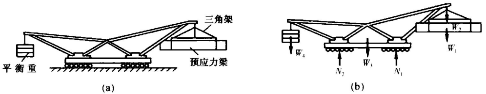
图 1-7 平面平行力系
