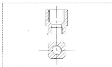
实例名称 实例63 绘制拉头 学习目的 掌握圆、矩形、图案填充命令的使用方法 视频长度 00:13:50 难易指数 ★★★★★ 所在页码 116
