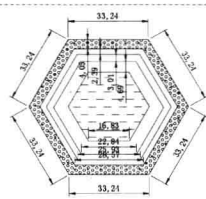
实例名称 实例120 标注喷泉结构图尺寸 学习目的 掌握线性、阵列命令的使用方法 视频长度 00:03:14 难易指数 ★★★★★ 所在页码 276
