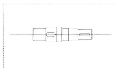
实例名称 实例69 绘制带键槽的轴 学习目的 掌握旋转命令的使用方法 视频长度 00:11:40 难易指数 ★★★★★ 所在页码 132
