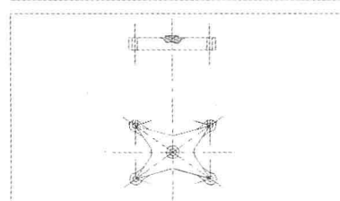
实例名称 实例72 绘制等强度梁 学习目的 掌握样条曲线、圆、直线命令的使用方法 视频长度 00:24:21 难易指数 ★★★★★ 所在页码 138
