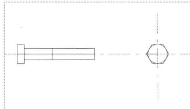
实例名称 实例57 绘制螺栓 学习目的 掌握多边形、偏移、圆命令的使用方法 视频长度 00:08:11 难易指数 ★★★★★ 所在页码 101
