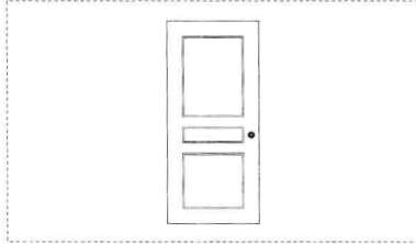
实例名称 实例165 绘制单开门立面图例 学习目的 掌握直线、偏移命令的使用方法 视频长度 00:03:25 难易指数 ★★★★★ 所在页码 366
