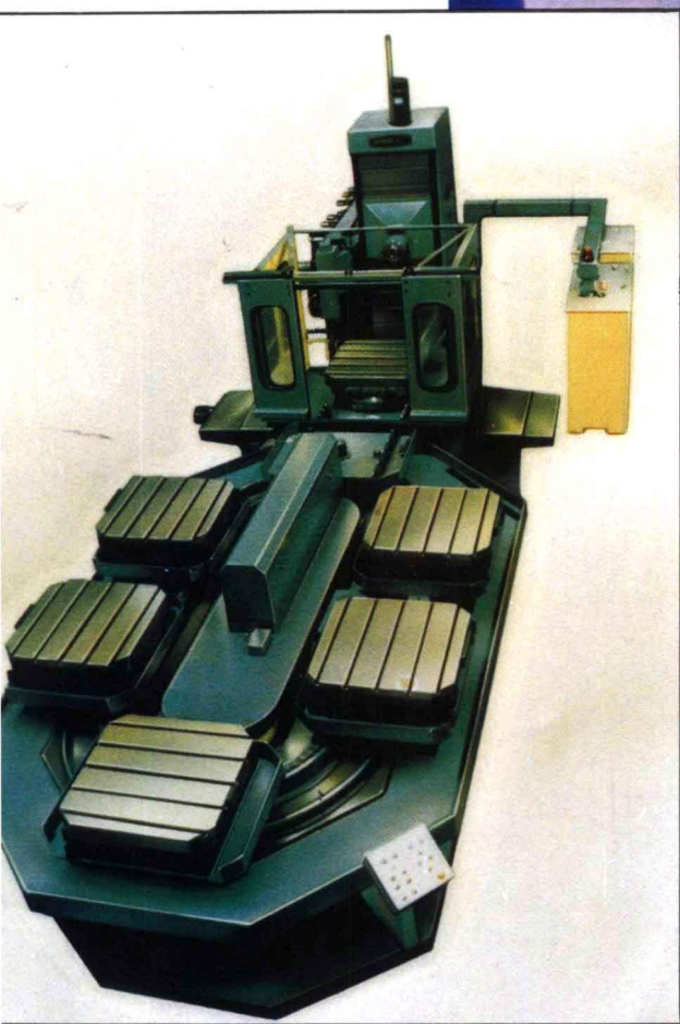
◁ 昆明机床厂最新研制的FMC-1000H 精密箱体柔性制造单元，是国家“七五”期 间重点科研攻关成果
