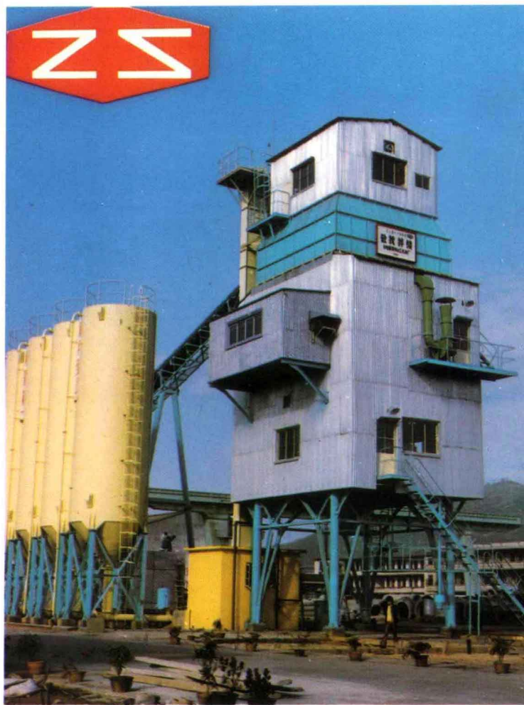
▷ 郑州水工机械厂制造的郑水牌自动化 混凝土搅拌楼
