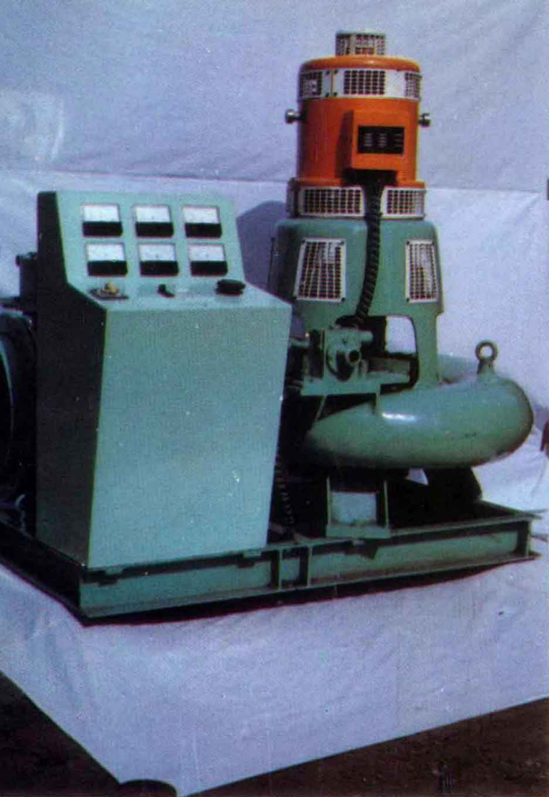
◁ 广西玉林水电设备厂生产的 8kW 微型整装机组
