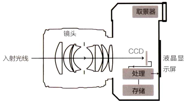
数码相机的光学原理图
