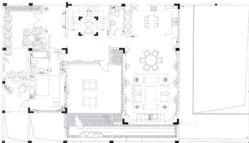
平面布置图
