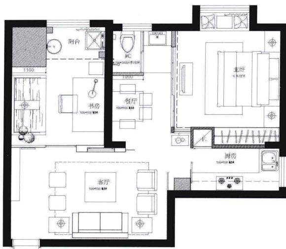
平面布置图
