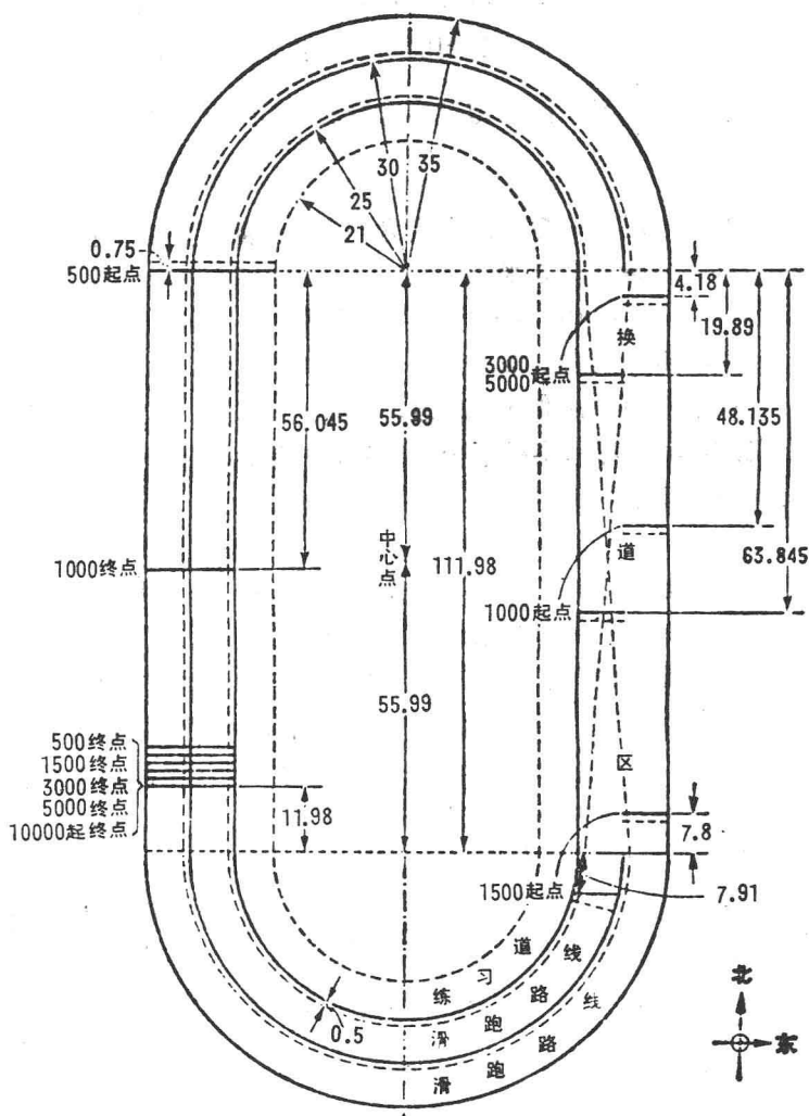
图一 速度滑冰400米标准场地平面图 (单位: 米)
