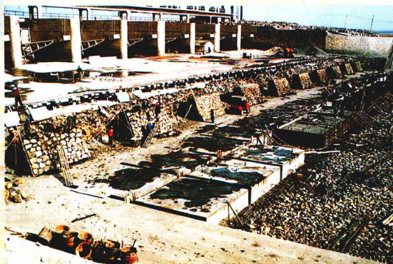
1999年泄洪闸加固工程
