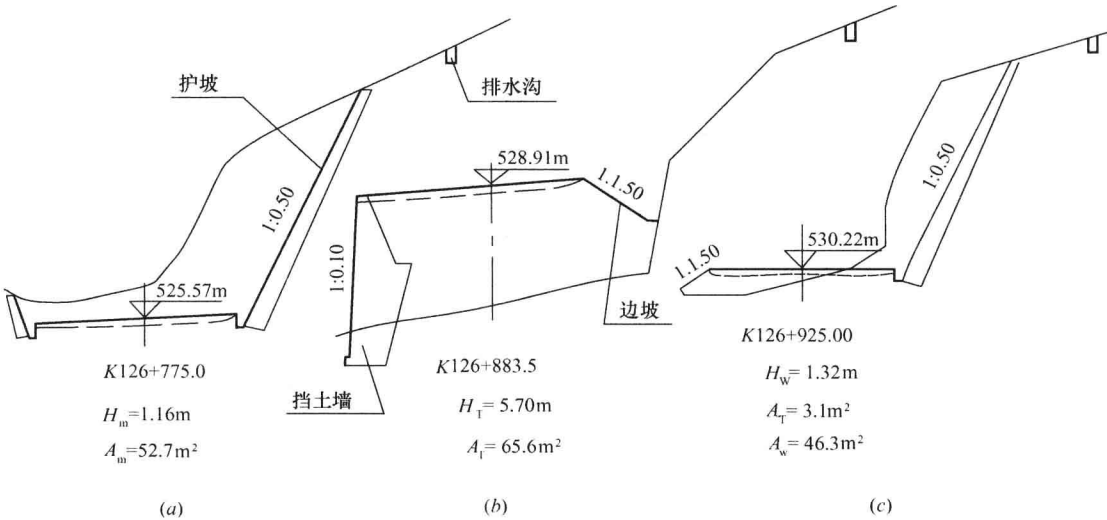
图2-2 路基横断面图
