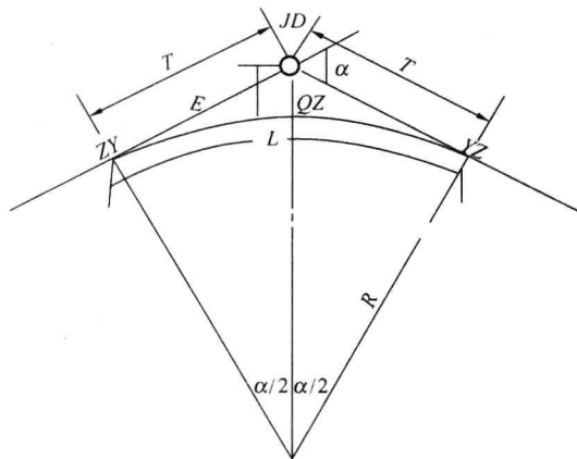
图 2-3 圆曲线要素示意图
