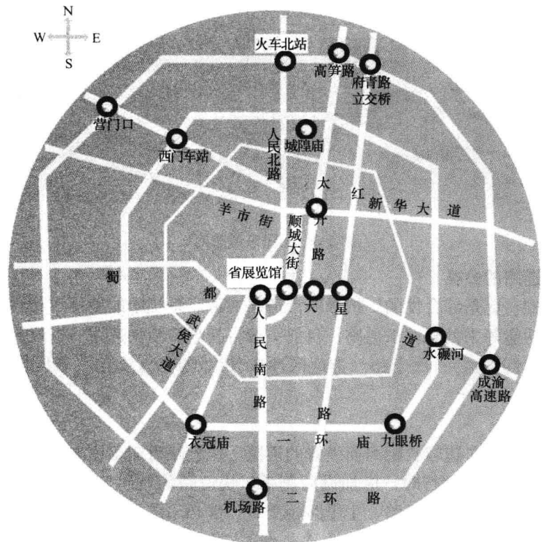
图 1-2 成都道路网
