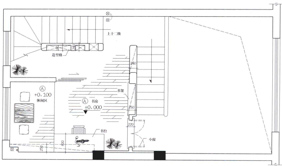
一层阁楼平面布局图
