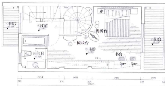
二层平面布局图
