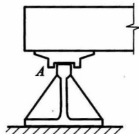
图 1.12 固定铰支座 (a)、(b) 固定铰构造; (c)、(d) 固定铰支座计算简图
