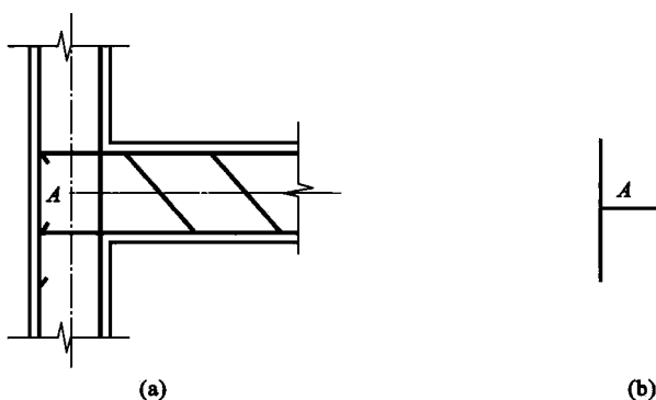
图 1.10 钢筋混凝土梁柱结点——刚结点 (a) 钢筋混凝土梁柱结点做法；(b) 刚结点计算简图
