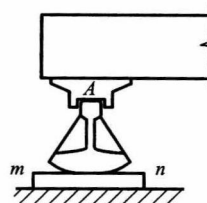
图 1.11 活动铰支座 (a) 桥梁活动铰支座; (b) 辊轴支座; (c) 摇轴支座; (d) 活动铰支座计算简图
