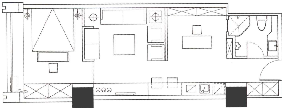
平面布置图
