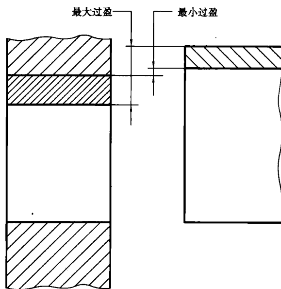
图 7 过盈配合
