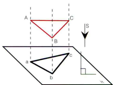
图1-2-2 正投影法
