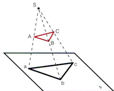
图1-2-4 中心投影法
