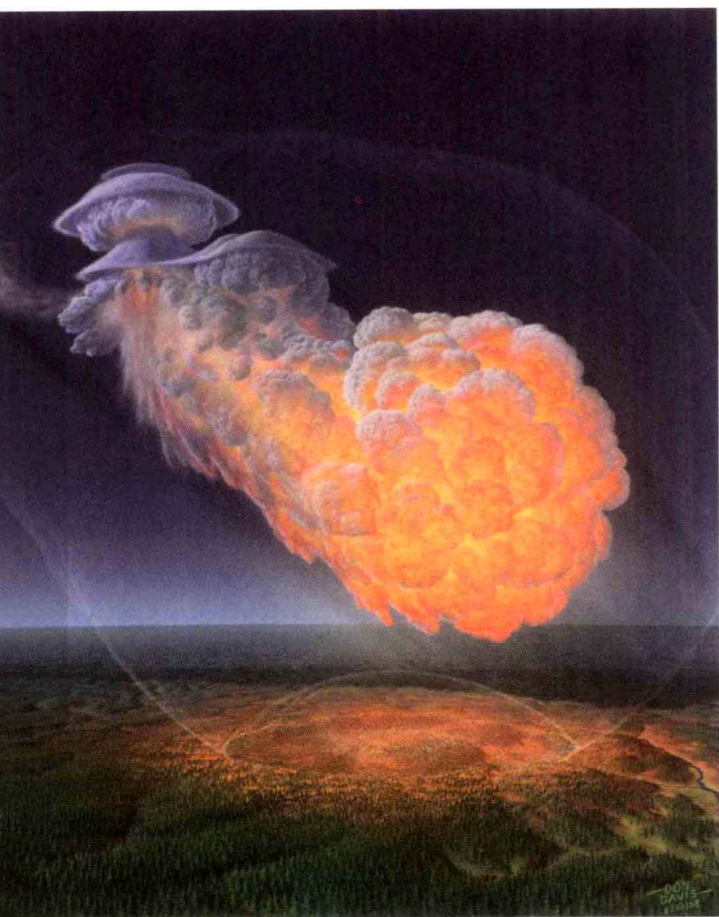
通古斯爆炸模拟图
