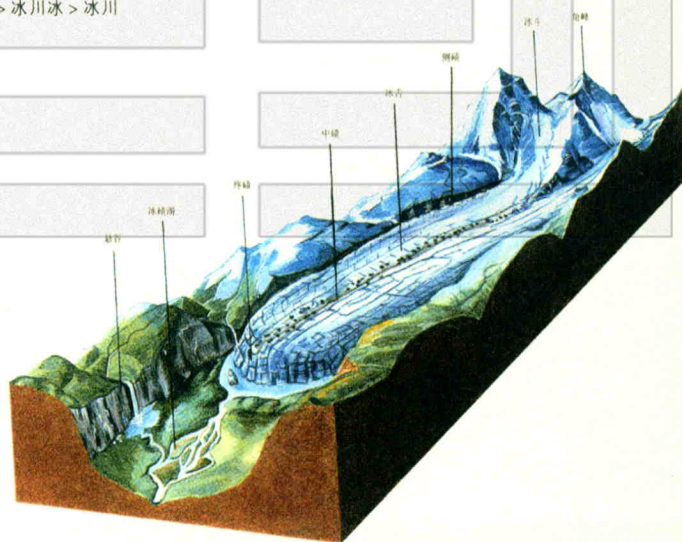
大型冰川 - 山谷冰川模式图
