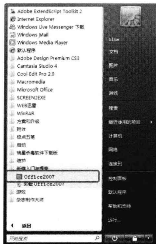
Windows 7 系统
