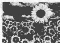
A. 绿色植物光合作用
