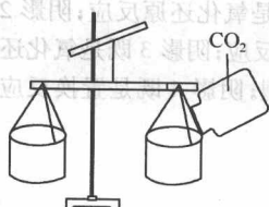
C. 测定 CO 2 的密度
