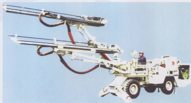
MERCURY-14型液压凿岩台车
