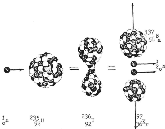
甲、核分裂反應次序
