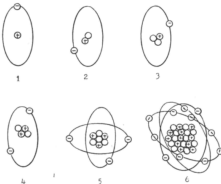
圖 1.1 典型的原子結構 (⊕：質子，⊖：電子，○：中子) [ 1：氫原子 ( A=1 , Z=1 )，2：氦原子 ( A=2 , Z=1 )，3：氦原子 ( A=3 , Z=1 )，4：氦原子 ( A=4 , Z=2 )，5：鋰原子 ( A=7 , Z=3 )，6：鈉原子 ( A=23 , Z=11 ) ]。
