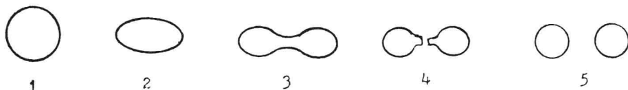
乙、核分裂的液滴模型
