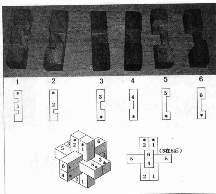
图1-5 / 孔明锁是中国古代建筑中的重要成就，它巧妙的结构关系体现了中国古人的聪明才智
