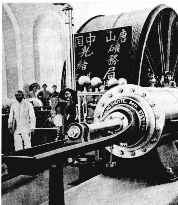
◎开滦早期使用的蒸汽绞车
