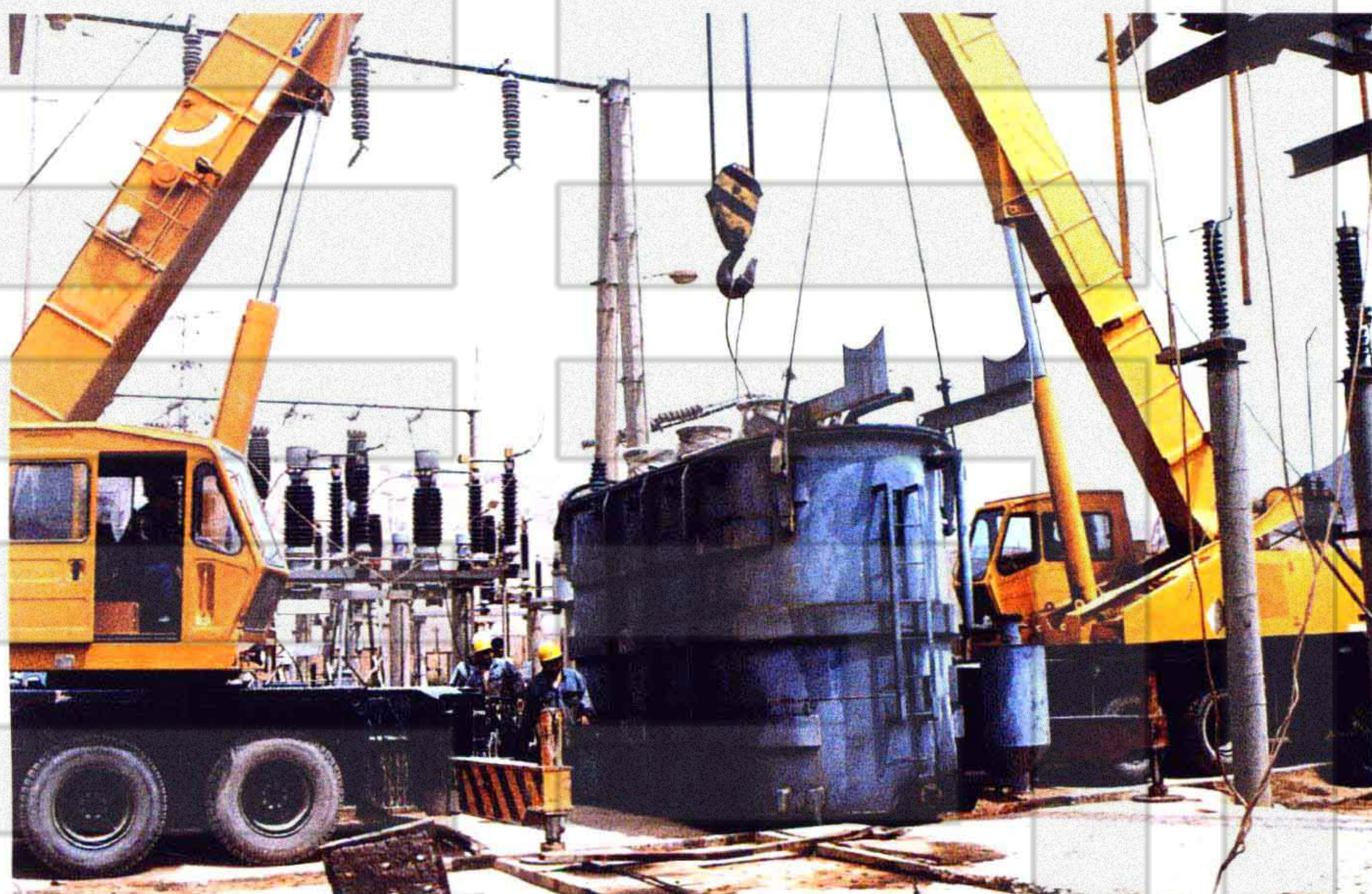
吐鲁番 110 千伏变电所 2 号主变就位
