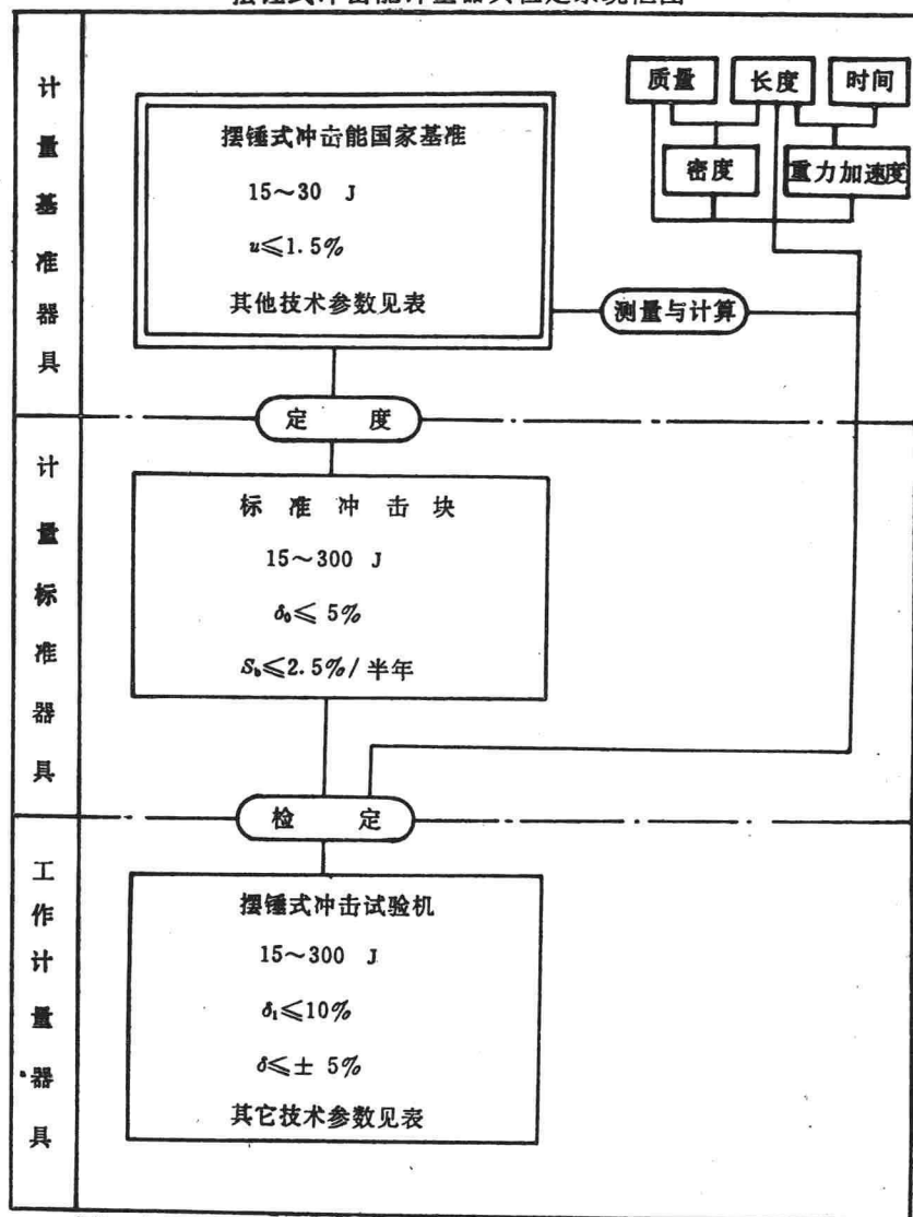
摆锤式冲击能计量器具检定系统框图
