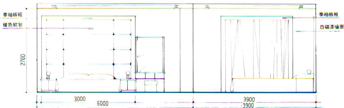
主卧室A立面图 1:30
