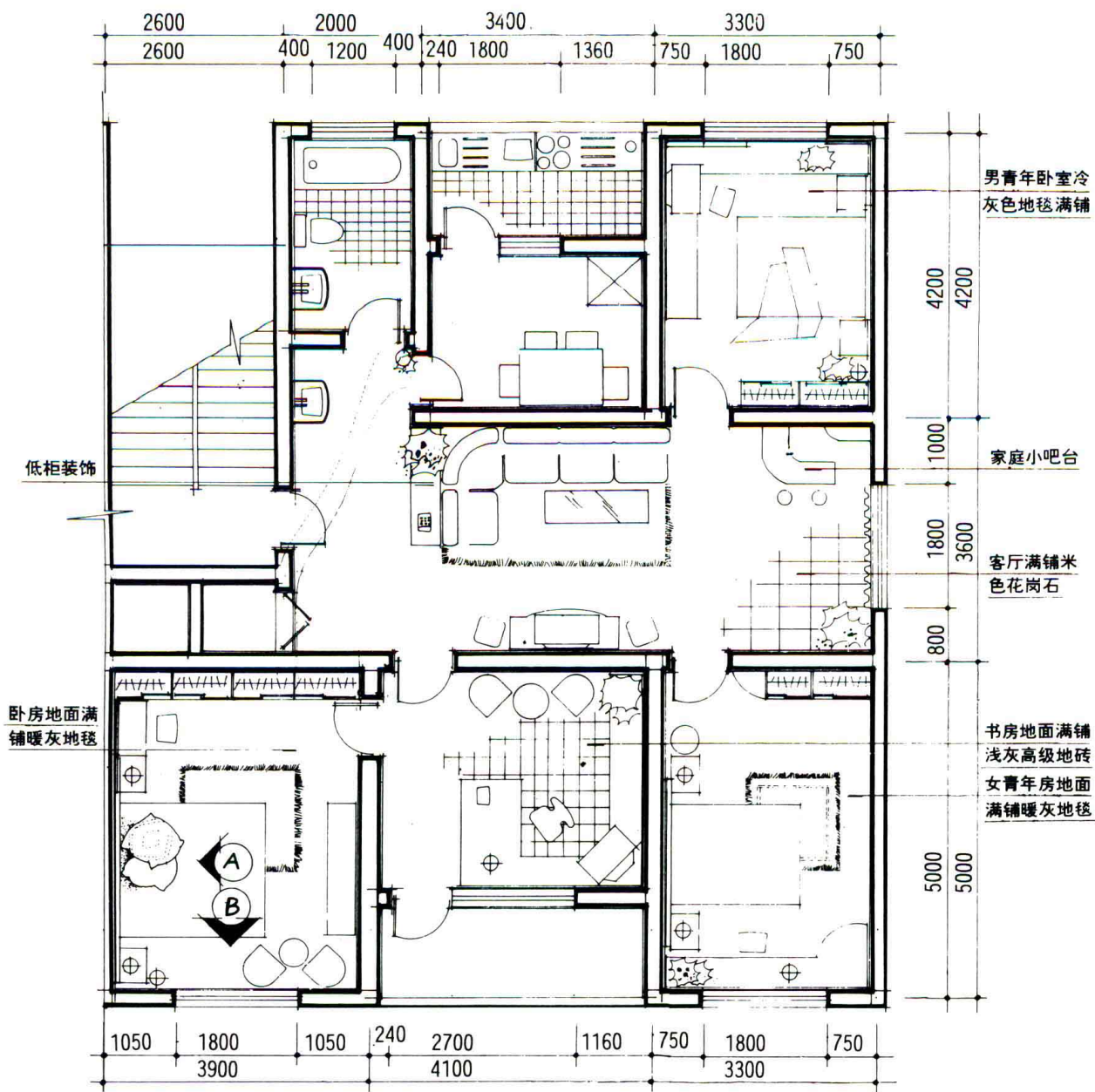
四室一厅平面图 1:50
