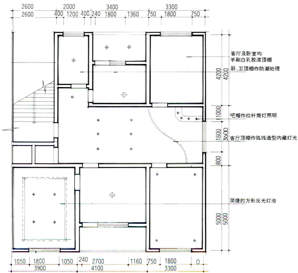
四室一厅顶面图 1:50
