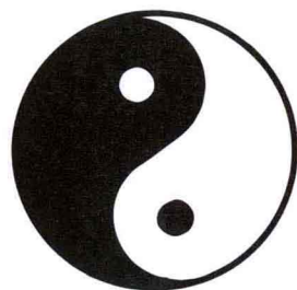
太极图
