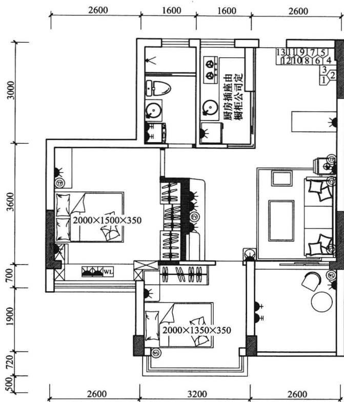
插座布置图
