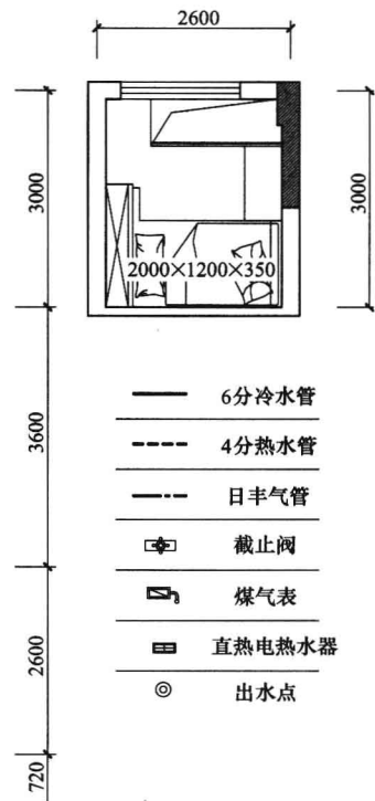
水路布置图
