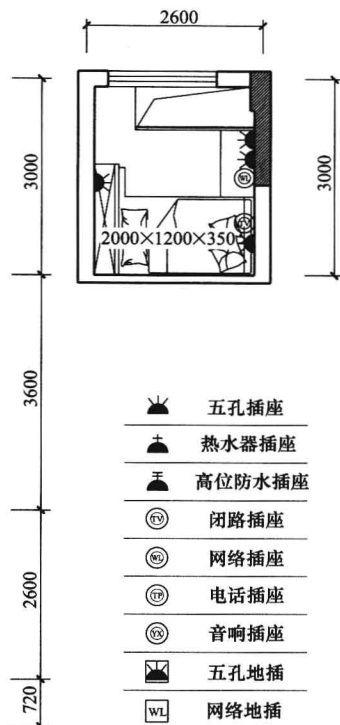
插座布置图
