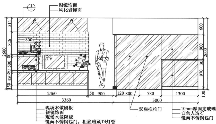
电视墙立面图
