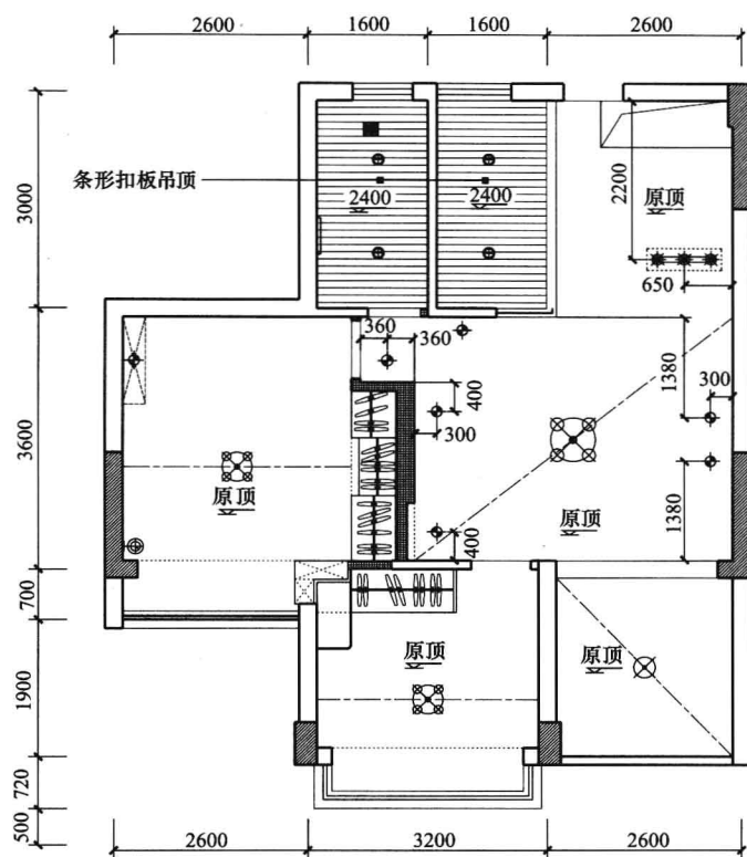
顶面布置图
