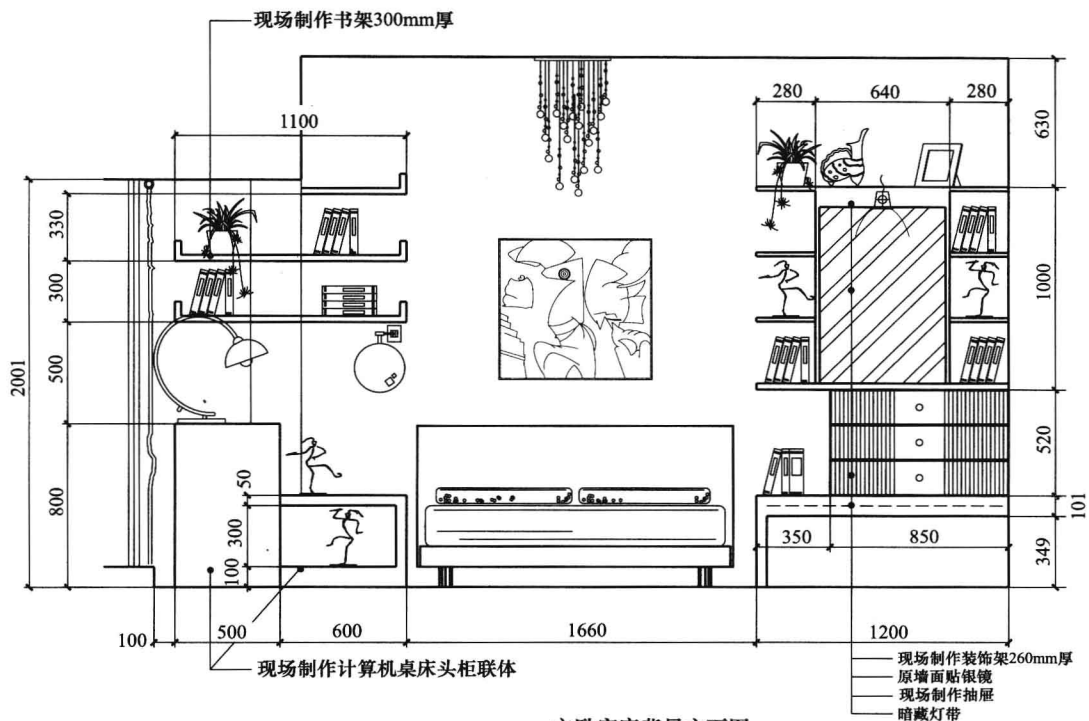
主卧室床背景立面图
