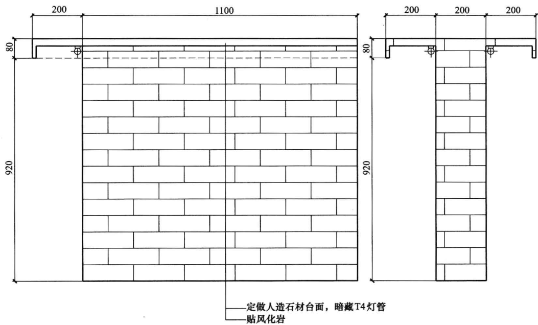
吧台尺寸放样图
