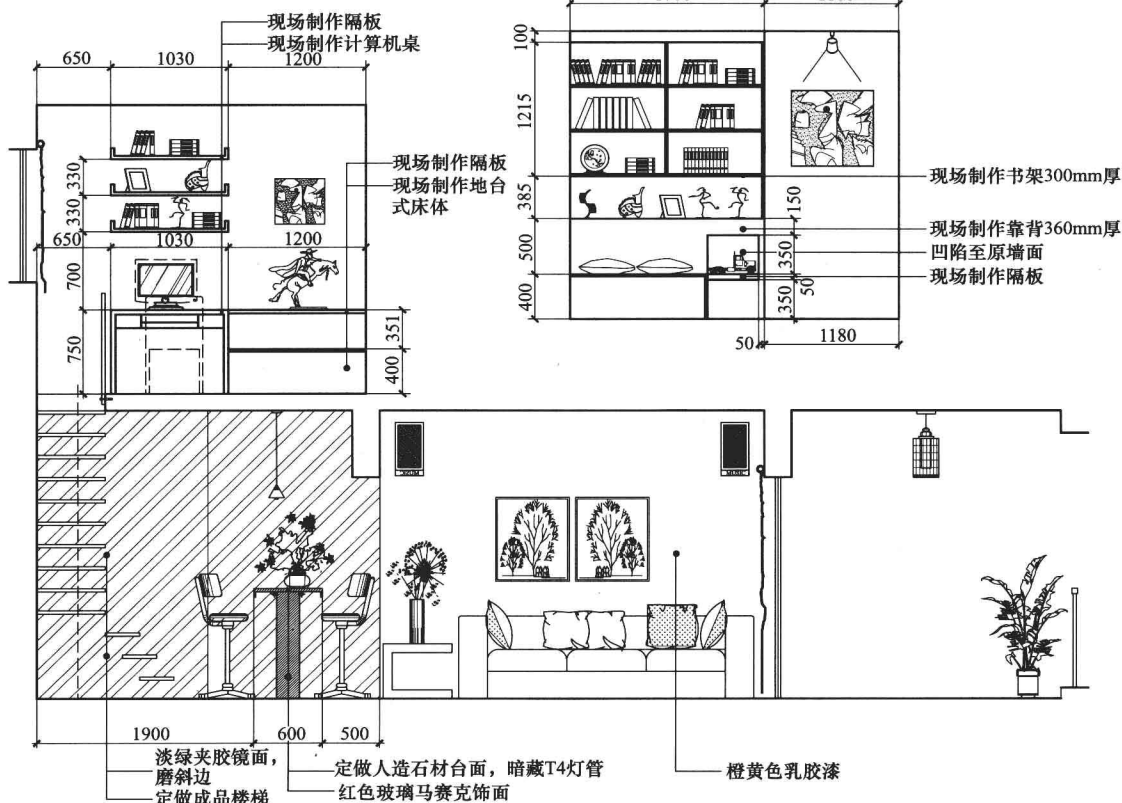
沙发背景立面图
