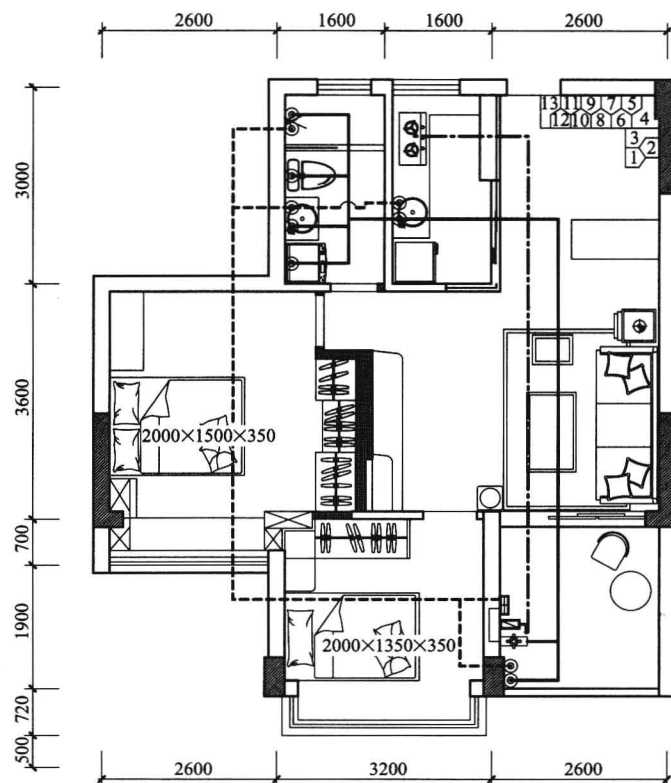
水路布置图
