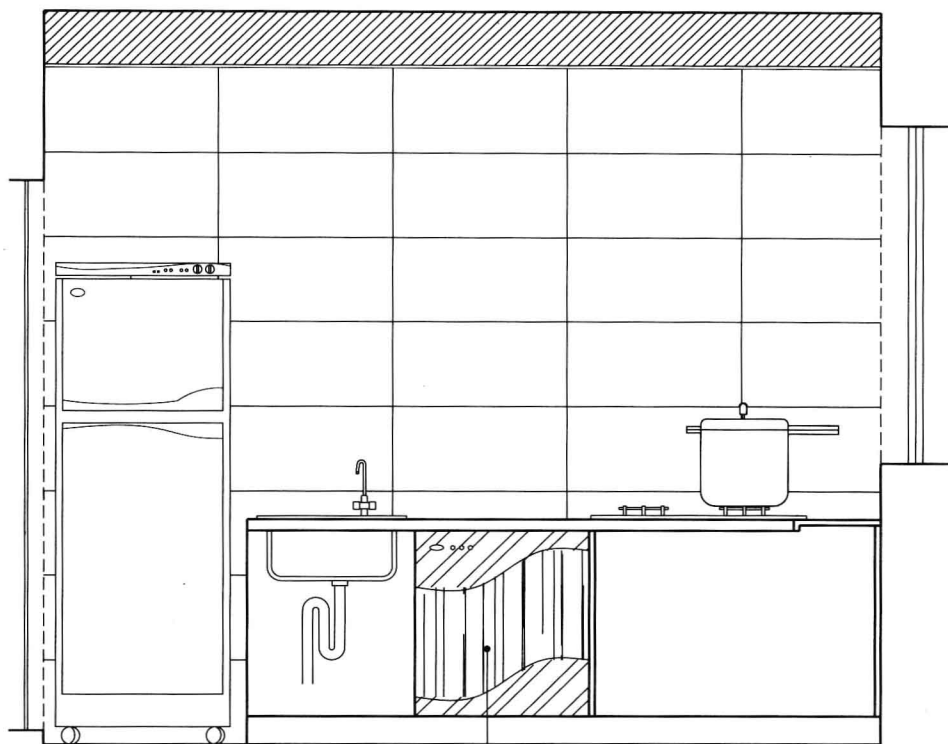
厨房立面图
