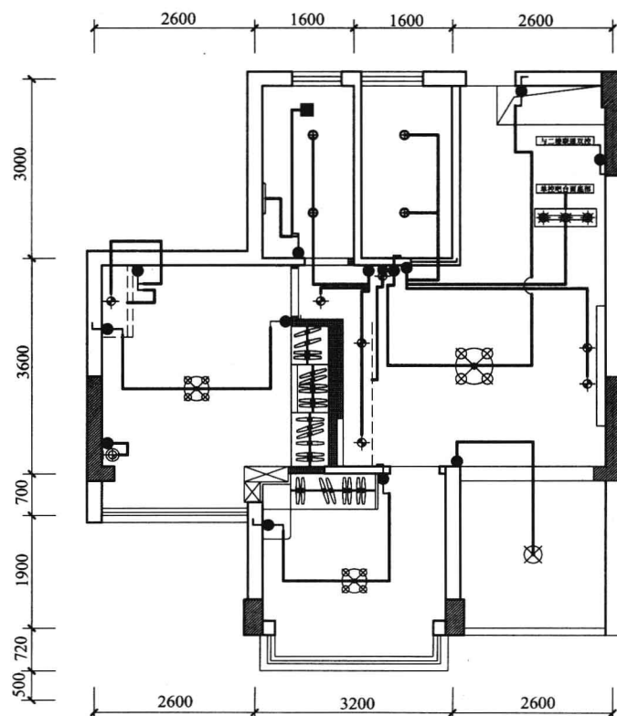
开关控制图
