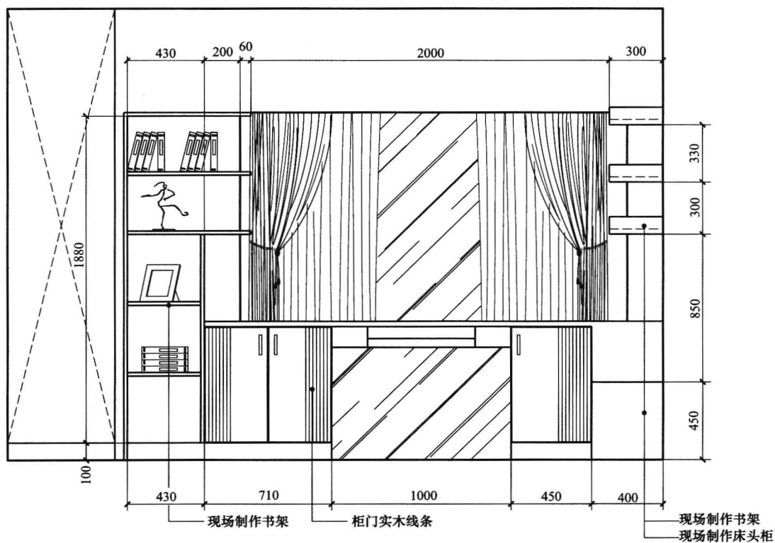
主卧室书桌立面图
