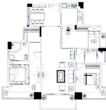
● 平面布置图
