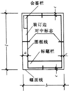
(c) A4 幅面
