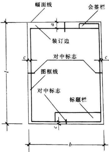
(b) A0~A3 立式幅面
