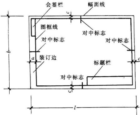
(a) A0~A3 横式幅面
