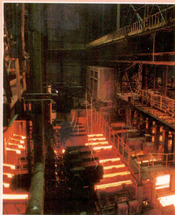
首钢自行设计制造安装的八流连铸机
