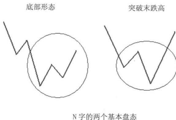
图 1-3 N 字突破的折线图
