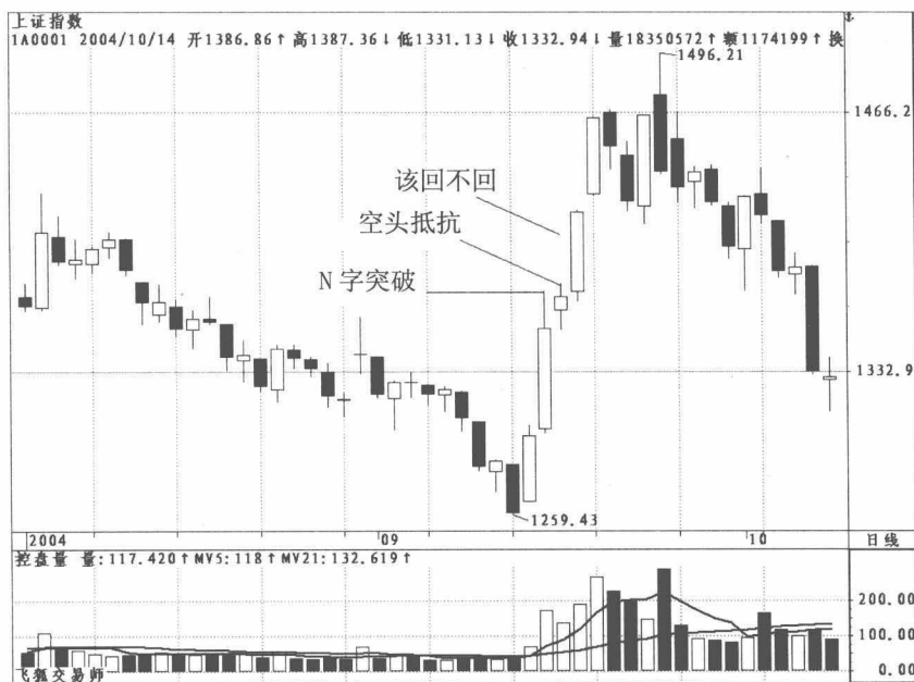
图 1-5 上证指数该回不回的 K 线图
