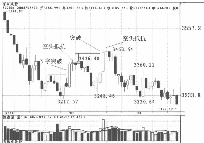
图 1-4 深证成指 N 字突破的 K 线图
