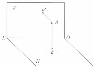
图 1-11 点的两面投影
