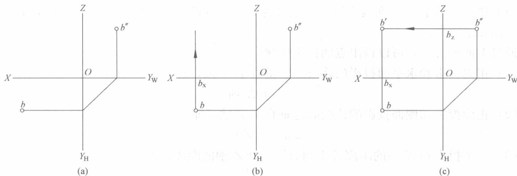
图 1-19 由点的 H 、 W 面投影求其 V 面投影
