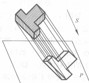
图 1-4 斜投影法
