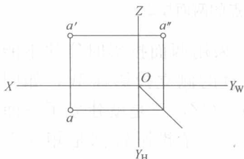
图 1-16 点的三面投影图
