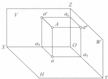
图 1-14 点的三面投影
