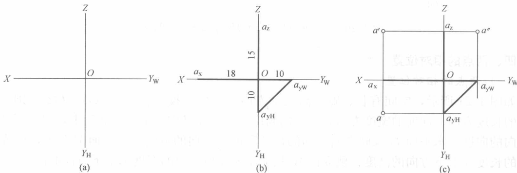
图 1-18 由点的坐标确定点的三面投影的位置
