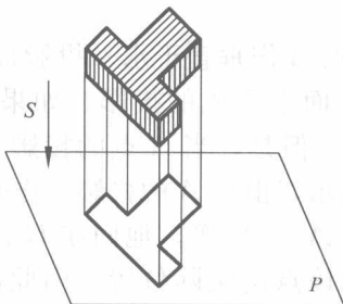
图 1-3 正投影法
