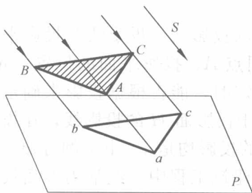
图 1-2 平行投影法
