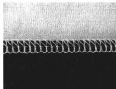
正面线迹
