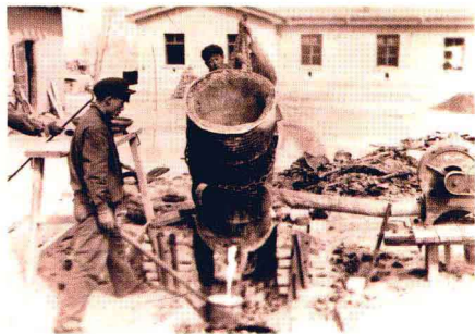
▲ 第一桶铁水(1958年6月)
