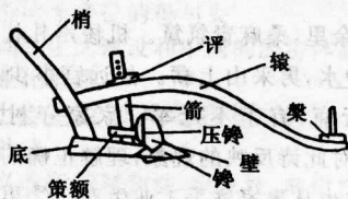
图3 曲辕犁详图
