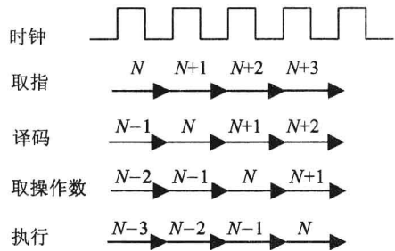
图 1-6 4 级流水线操作图
