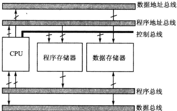
图 1-4 基本哈佛(Havard)结构
