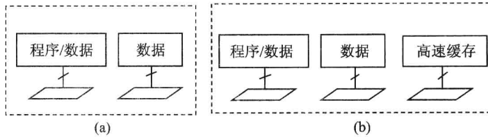
图 1-5 改进的哈佛结构
