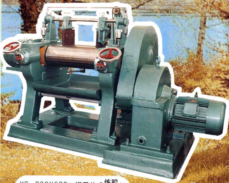
XS—230X630二辊开放式炼胶压延机
