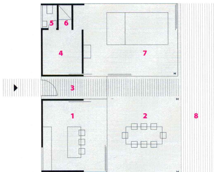
一区底层平面图
