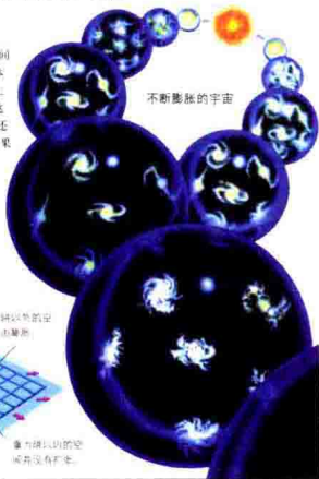
河外星系的
