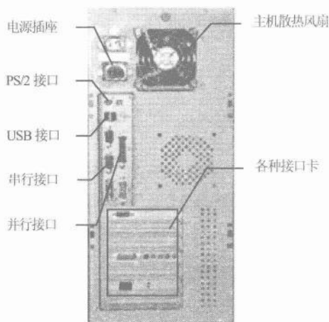
图 1-3 电脑主机的背面构成
