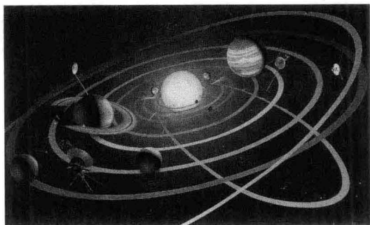
太阳系的运行图
