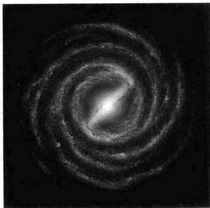
银河系的正面图
