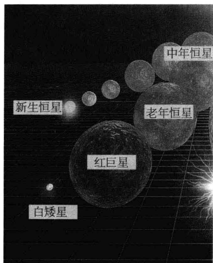
中小恒星的演化
