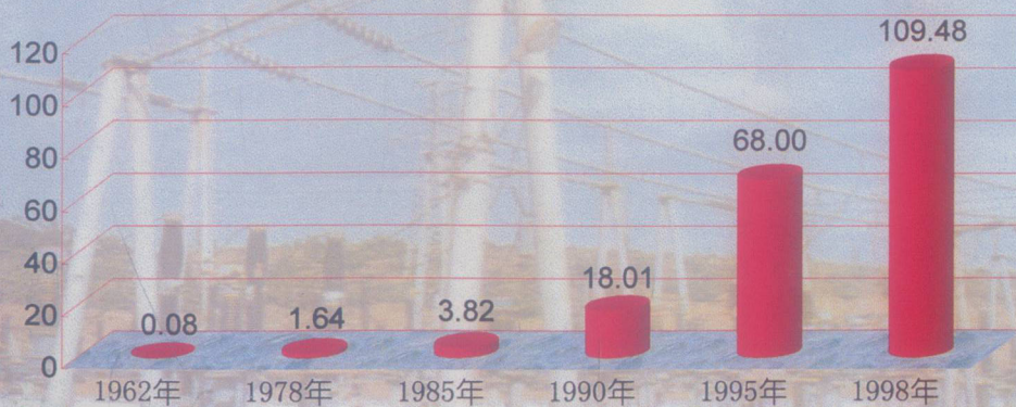
总发电量(亿千瓦时)
