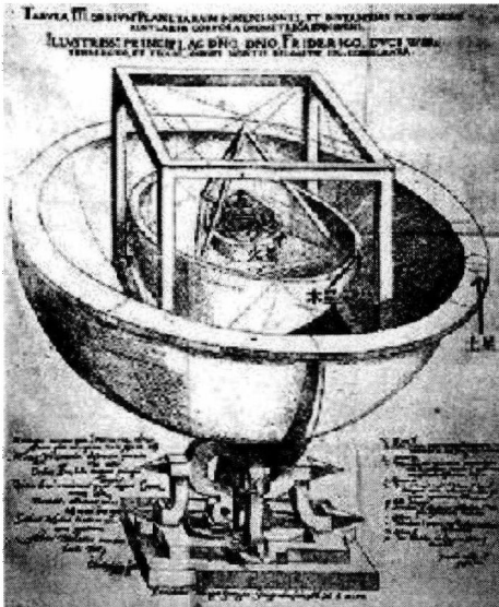
哥白尼的宇宙模型
