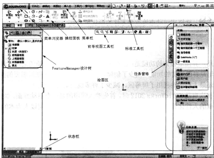
图 1-2 SolidWorks 2012 界面
