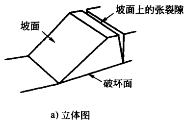
题 1-22 图 直线滑坡稳定系数计算
