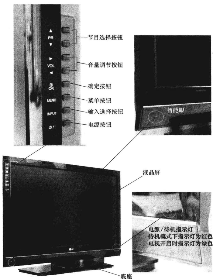
图 1-1 液晶电视前面板
