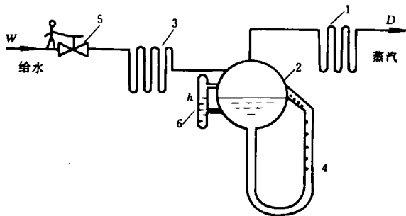
图 1-1 锅炉给水人工调节示意图
