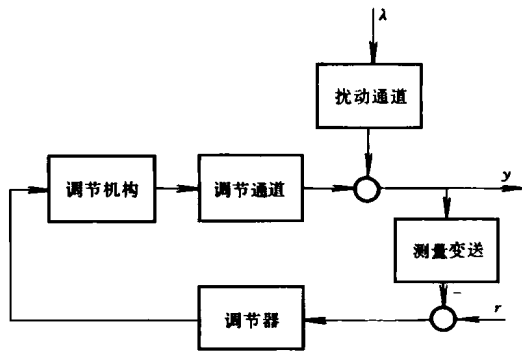
图 1-3 反馈控制系统
