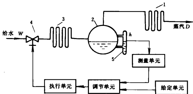
图 1-2 汽包锅炉给水自动调节示意图
