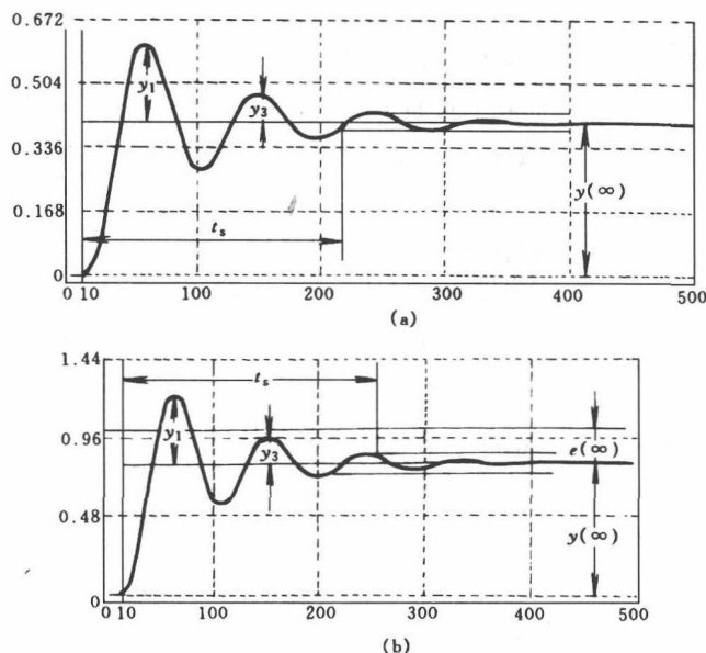
图 1-8 控制过程曲线
