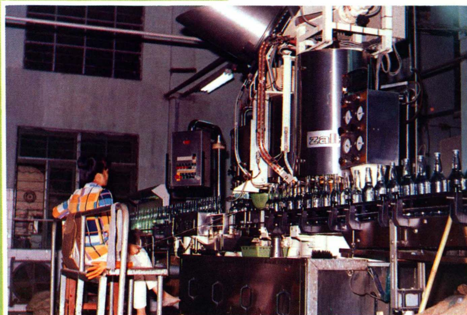
佛山市石灣酒廠引進 的西德米酒自動灌裝綫
