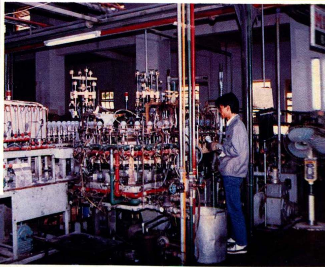
佛山市電器照明公司引進 日本的東芝MS普泡裝配生產綫
