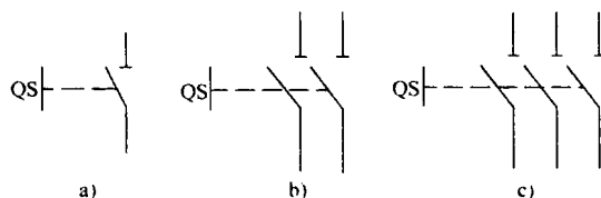
图 1-2 刀开关图形符号
