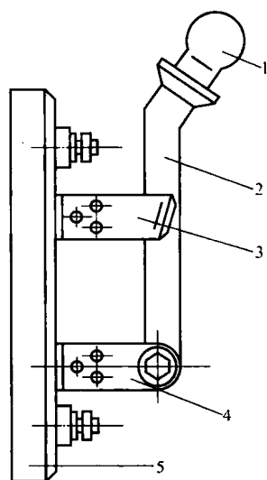
图 1-1 刀开关结构
