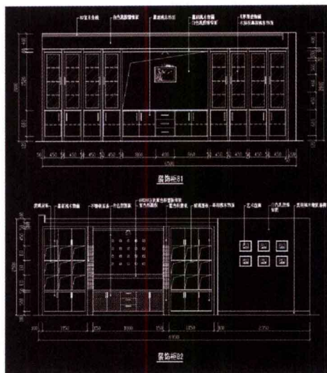
CAD立面图
