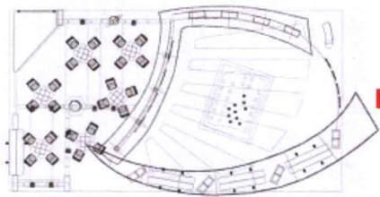
展示方案CAD平面图
